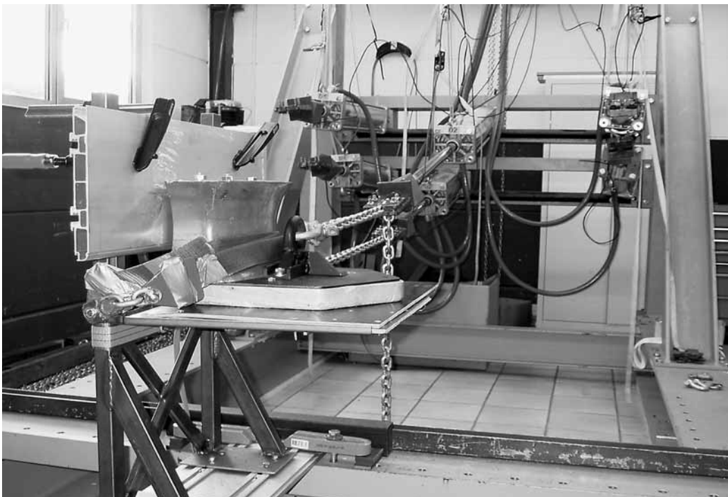
SAFETY-Sitze längs
